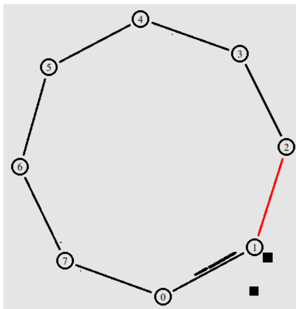
Εικόνα 5 – Αναπαράσταση της διακοπής ζεύξης μεταξύ 1 και 2
