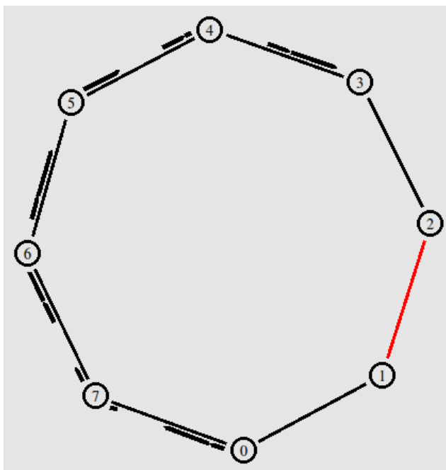
Εικόνα 6 – Αναδρομολόγηση των πακέτων της ζεύξης 0-3
