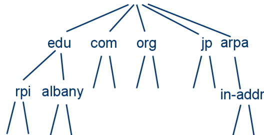
Σχήμα 1: Ιεραρχία DNS
